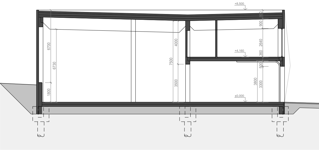
ŘEZ OBJEKTEM
