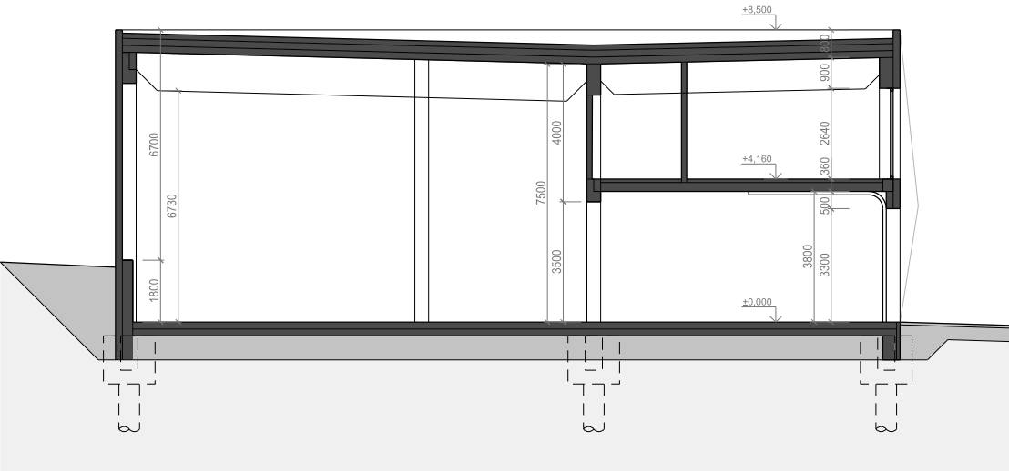
ŘEZ OBJEKTEM
