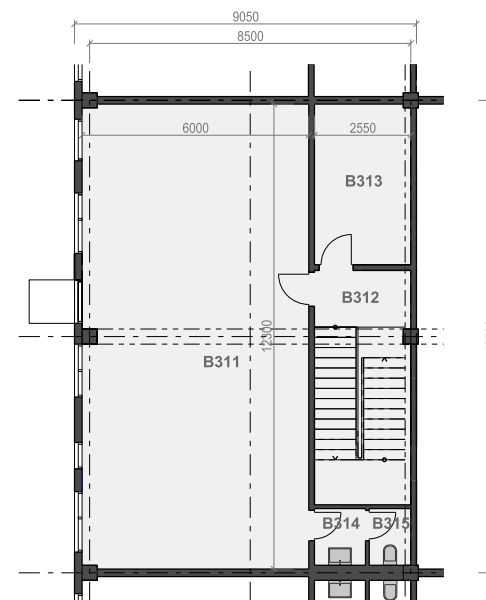
PŪDORYS 2.NP
