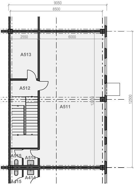
PŮDORYS 2.NP
