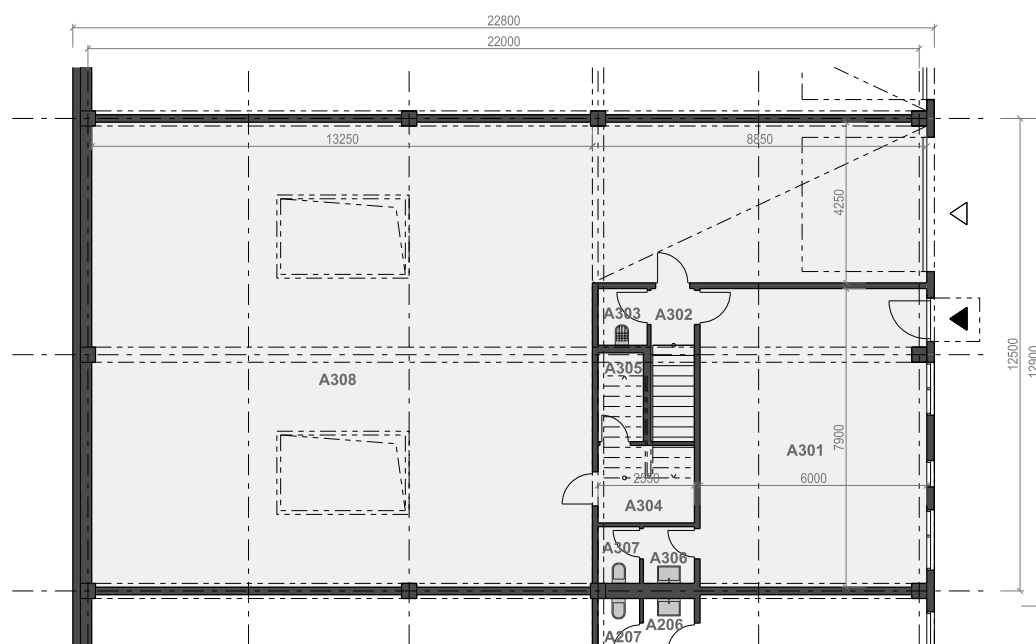
PŪDORYS 1.NP
