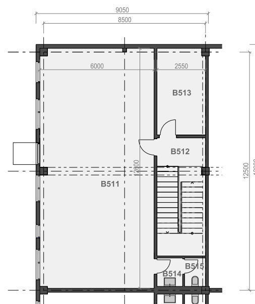
PŪDORYS 2.NP
