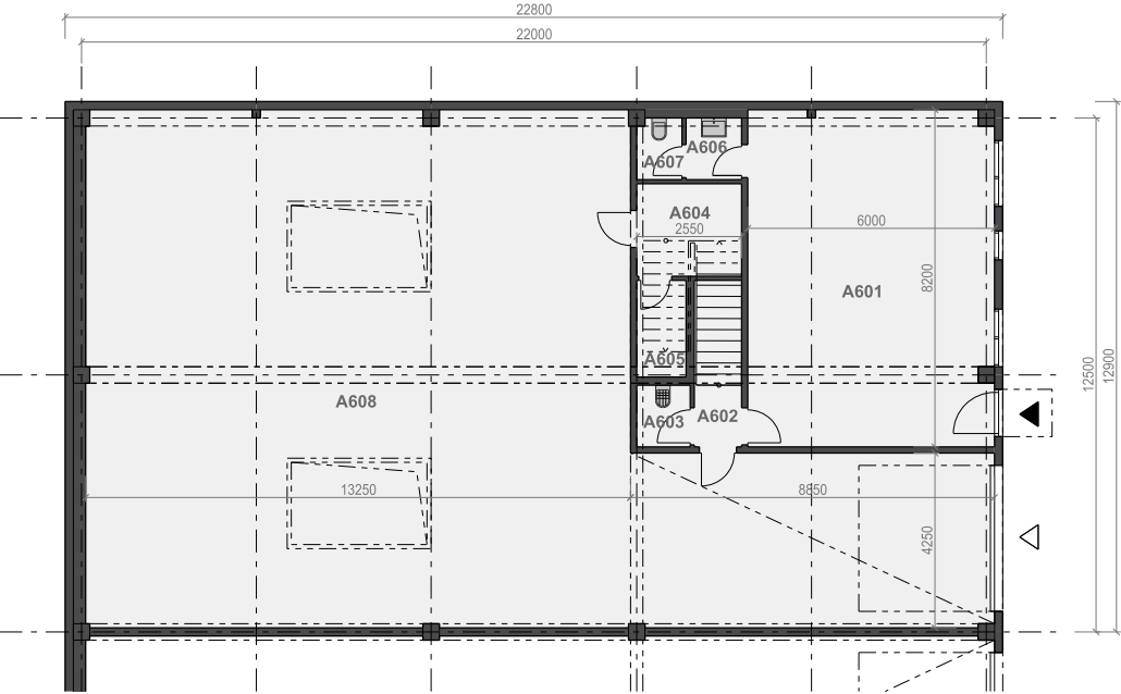
PŮDORYS 1.NP
