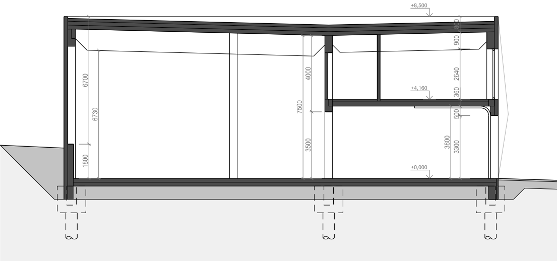
ŘEZ OBJEKTEM
