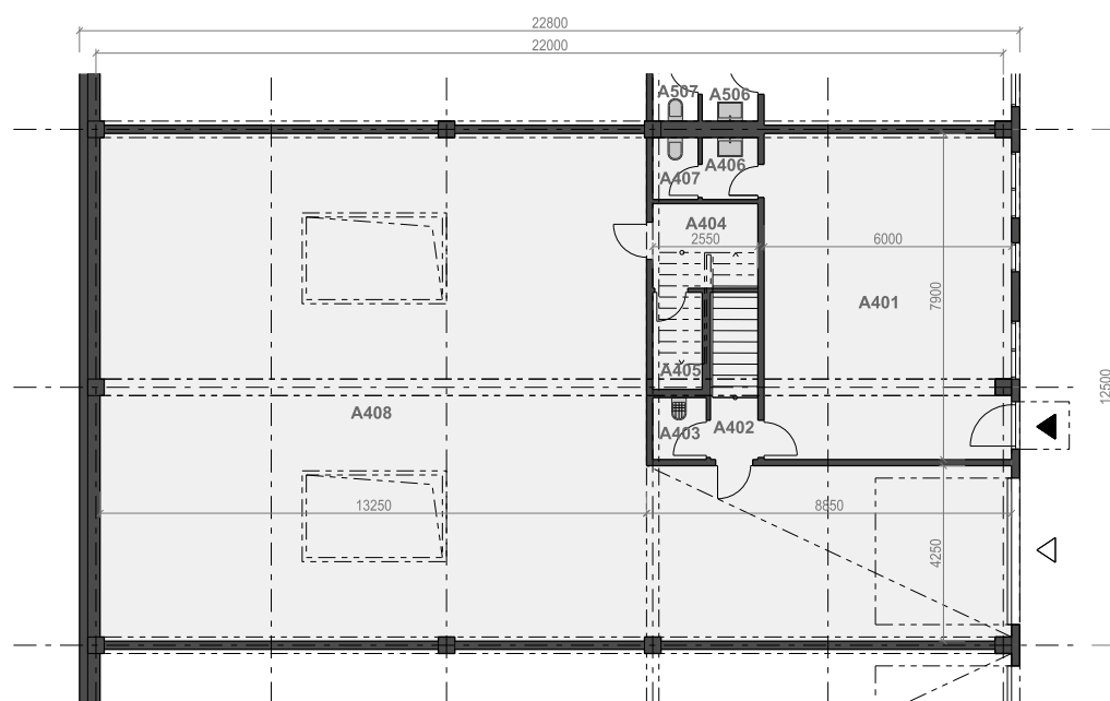
PŪDORYS 1.NP
