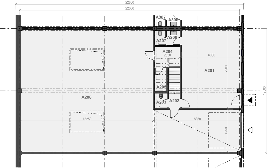
PŮDORYS 1.NP
