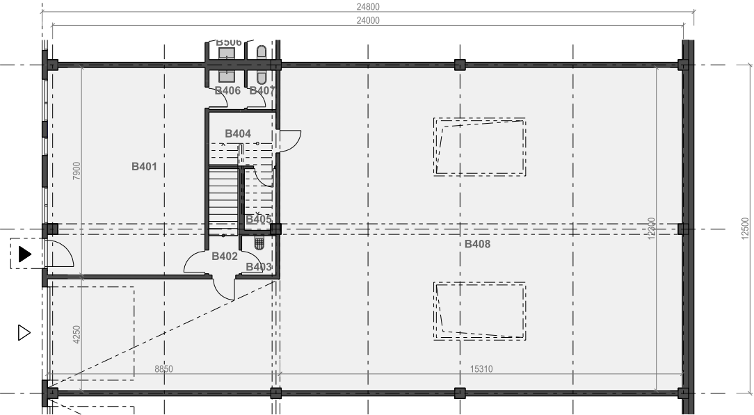
PŮDORYS 1.NP
