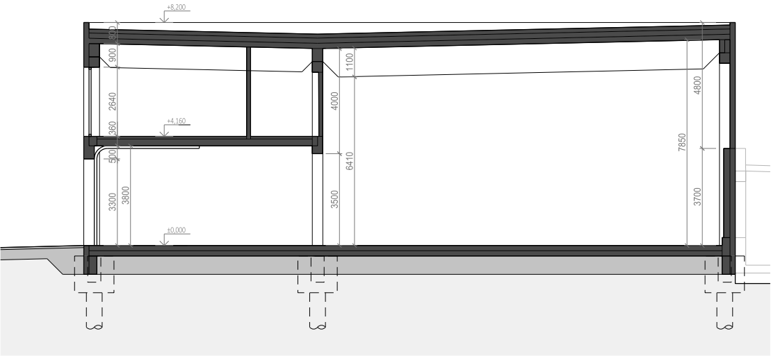
ŘEZ OBJEKTEM
