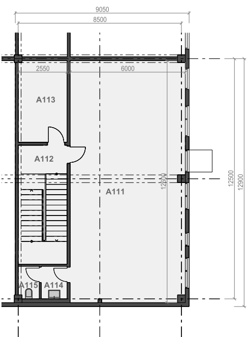
PŮDORYS 2.NP
