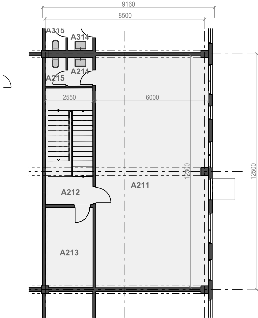
PŮDORYS 2.NP
