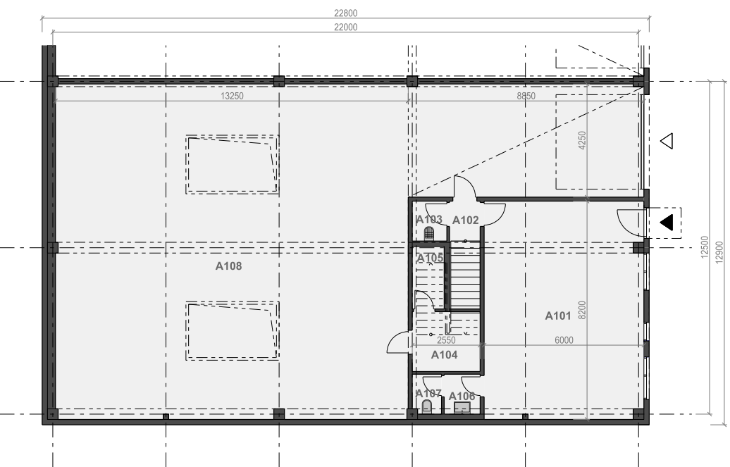
PŮDORYS 1.NP
