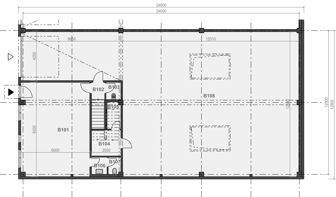
PŮDORYS 1.NP
