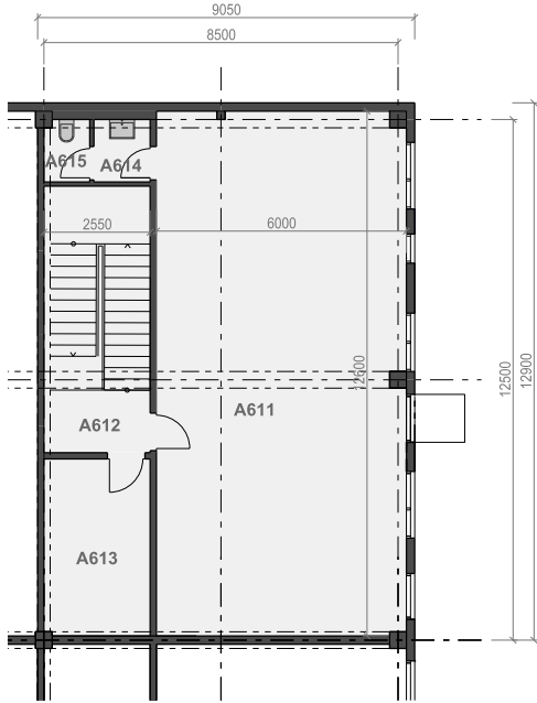
PŮDORYS 2.NP
