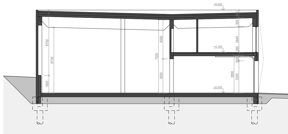
ŘEZ OBJEKTEM
