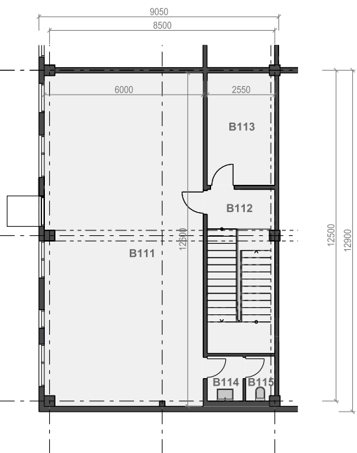
PŮDORYS 2.NP
