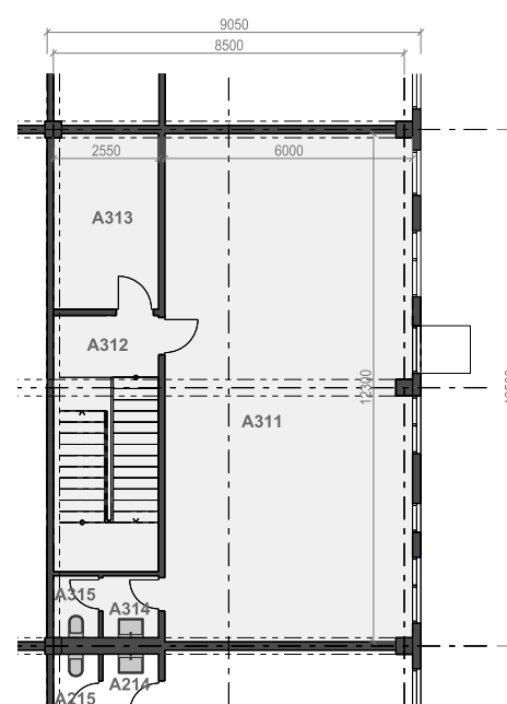
PŪDORYS 2.NP
